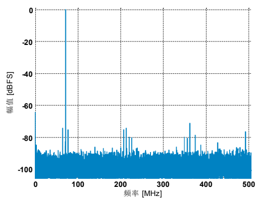
图 3: ADQ12DC-4C: 71 MHz.
